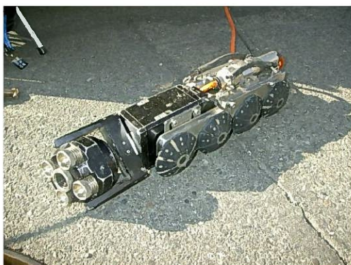
自社のTVカメラ調査車両
